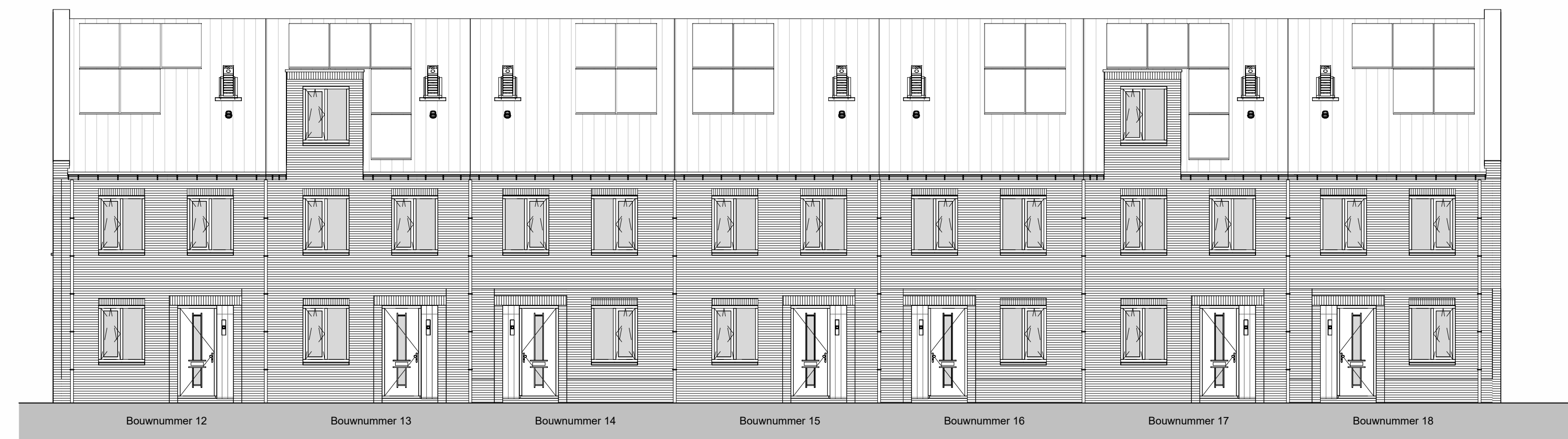
basisschema 1:100
